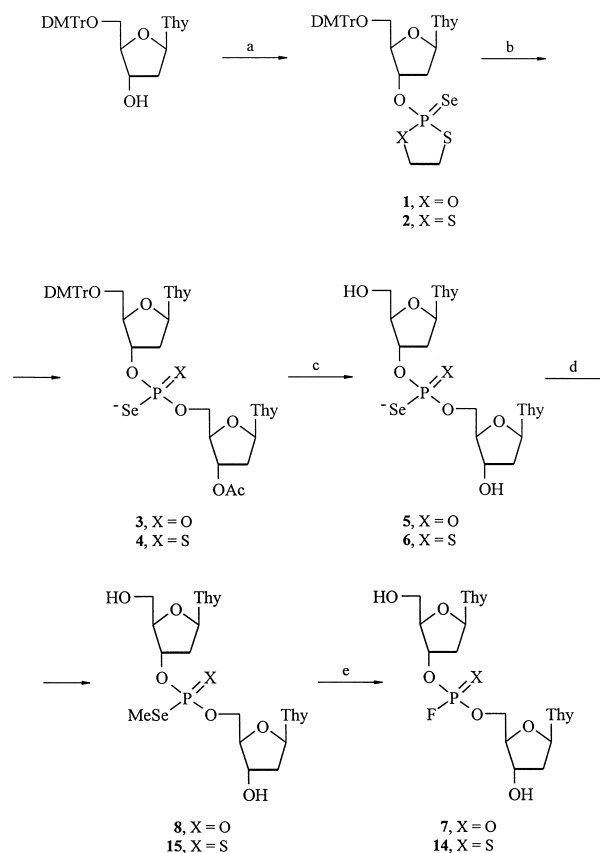
Scheme 1. (a) (i) N,N -diisopropylamino-1,3,2-oxathia(dithia)phospholane, 1 H -tetrazole; (ii) Se 8 ; (b) 3'- O -acetylthymidine, DBU; (c) (i) CH 3 COOH, (ii) NH 4 OH; (d) MeI; (e) AgF for 8 , Et 3 NHF for 15 .
